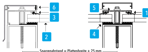
Verbindungsprofil
