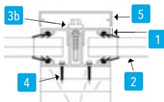
Randprofil
