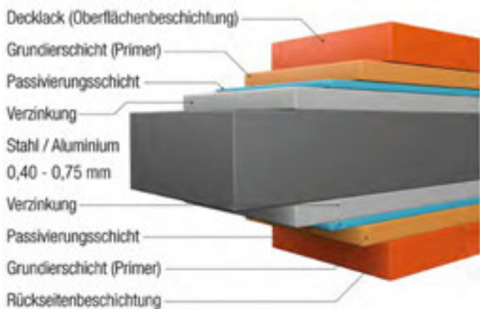
Beispiel: Beschichtungsaufbau
