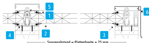
Verbindungsprofil
