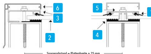
Verbindungsprofil
